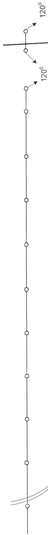
Prilog 1: Uzdužni profil dionice dalekovoda
